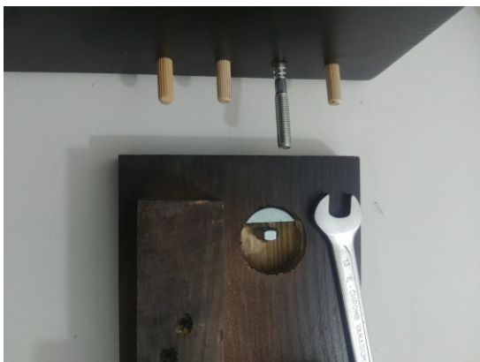
Соедините детали согласно отверстий и зажмите гайку
